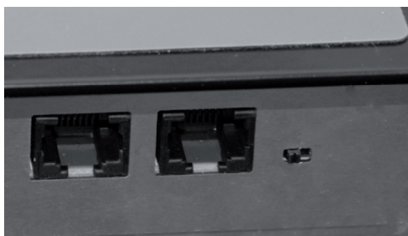
RCC-03-Terminierung aktiviert (Linksstellung)
