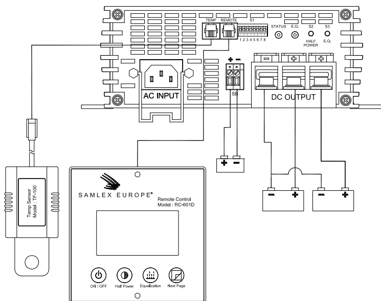
Schéma 5b Réaliser des Branchements WSC-1230SB Li
