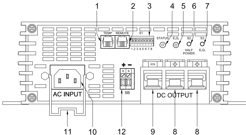
Schéma 1b Chargeur WSC-1230SB Li Vue de Face
