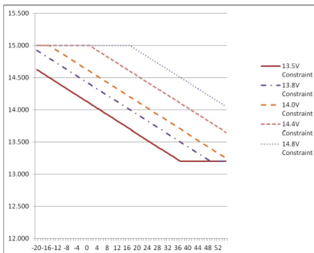
Schéma 17 Compensation de Température pour Modèle 12V
