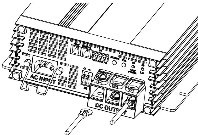
Schéma 6 Installation des Câbles WSC-1230Li / WSC-1230SB Li
