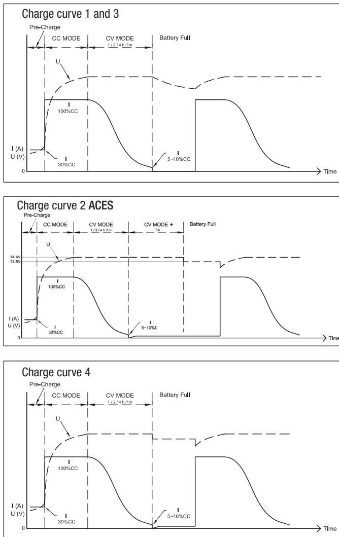
Schéma 19 Caractéristique de Charge
