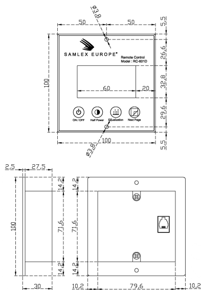
Schéma 13 Télécommande RC-601D Dimensions (mm)
