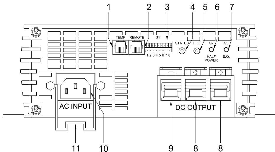
Schéma 1a Chargeur WSC-1230Li Vue de Face
