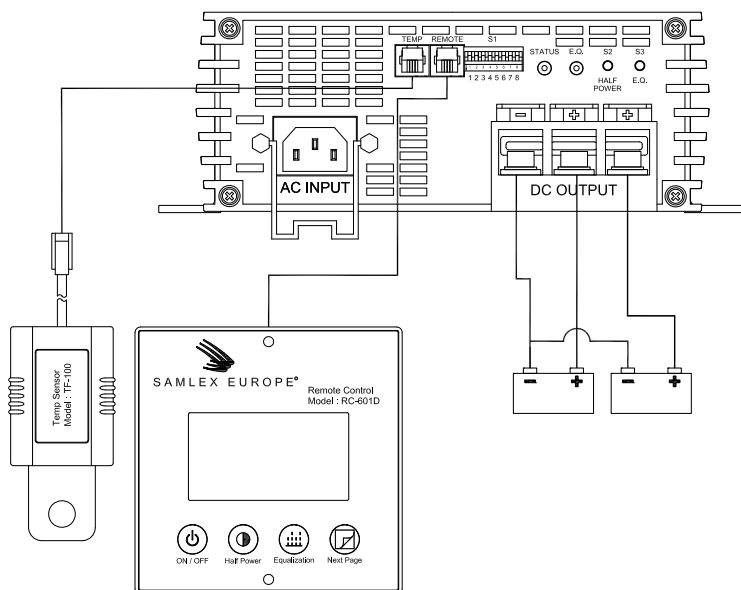
Schéma 5a Réaliser des Branchements WSC-1230Li
