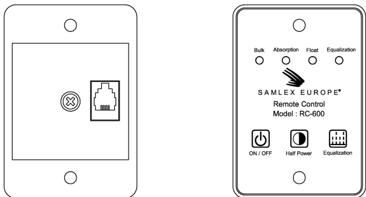
Schéma 10 Télécommande RC-600
