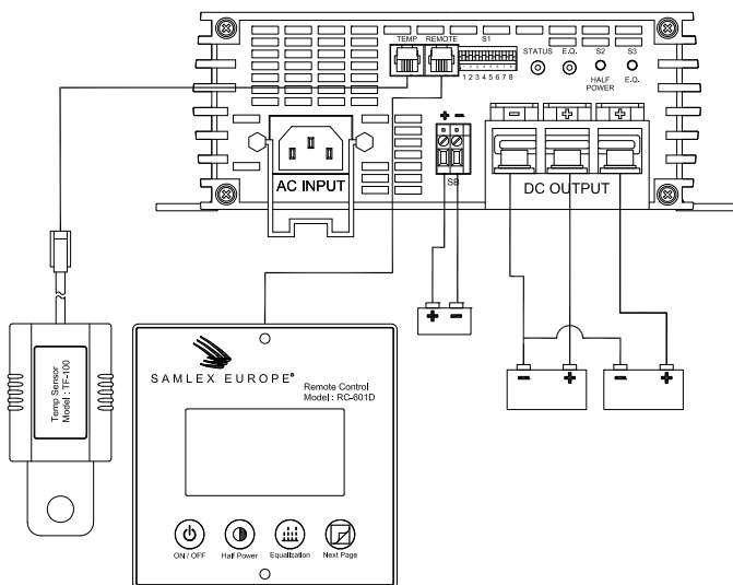
Schéma 14b Réaliser des Branchements du RC-601D au WSC-1230SB Li
