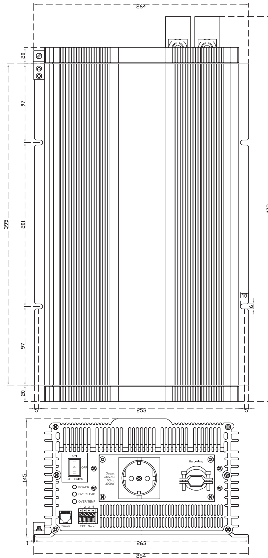
Fig. 8.1: Dimensiones generales y ranuras de montaje de SWI 3000.
