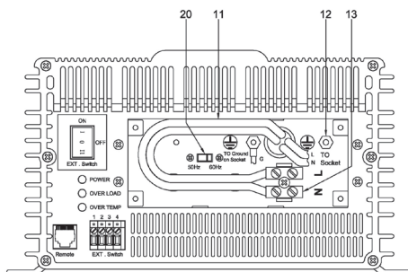
Fig. 6.1 (b) SWI 3000, Trasera - Mostrando compartimento con terminales para cableado.
