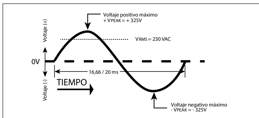
Fig. 5.1: Forma de onda sinusoidal pura 230 VAC, 50 / 60 Hz.
