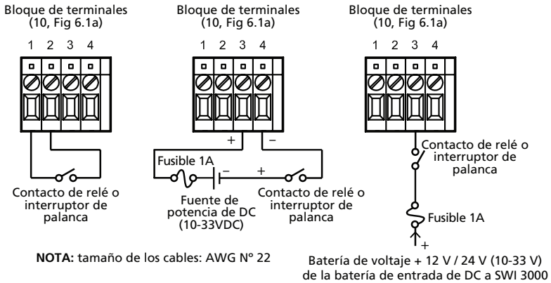
Fig. 8.2(a) – Cable-2 del Control ON / OFF usando contacto del interruptor / relé
