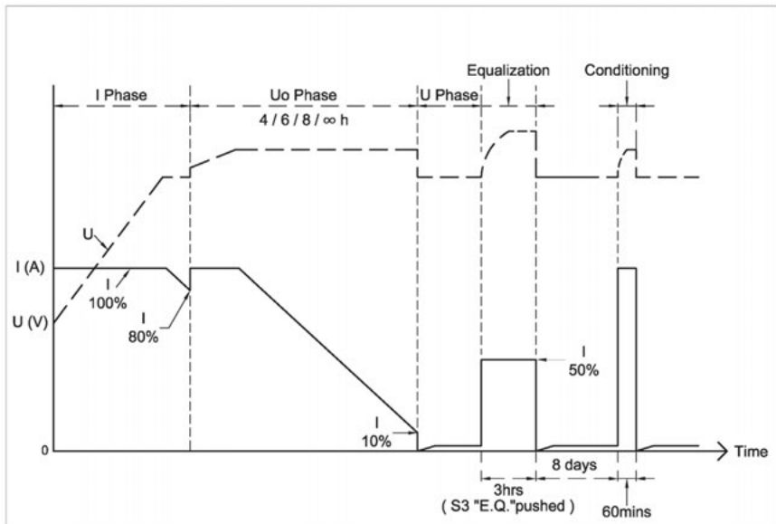
Afbeelding 19 Laadkarakteristiek
