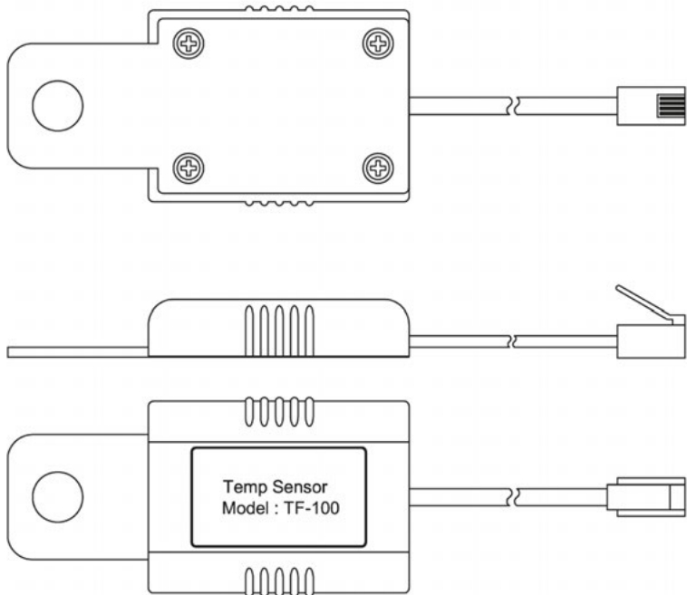
Afbeelding 12 Temperatuursensor TF-100
