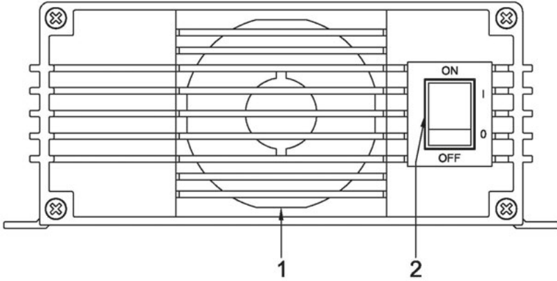
Afbeelding 3 Lader achteraanzicht
